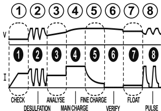
Fazy ładowania PULSE-TRONIC.
