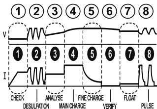
Fáze nabíjení PULSE-TRONIC.
